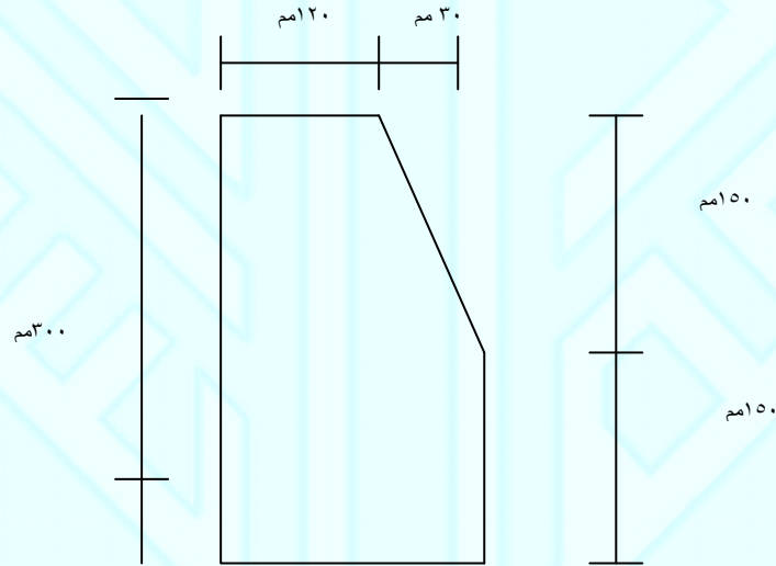
الشكل رقم ( ٢ ) مقطع عرضي لقالب جانبي
