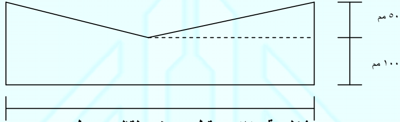
شكل رقم (١) : مقطع عرضي لقالب وسطي
